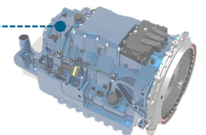
Mild-hybrid
