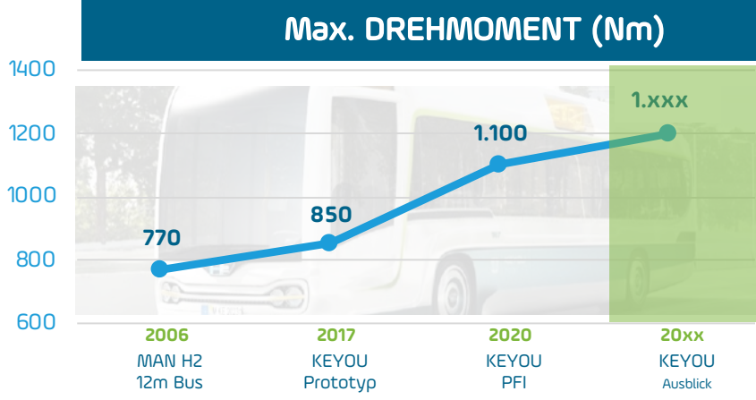
Beispiel 12m Bus: DEUTZ TCG 7.8 H2 mit KEYOU-inside
